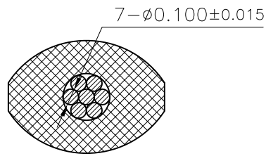
SECTION A-A (4:1)
