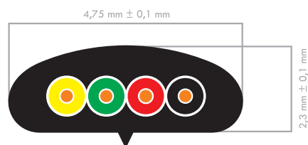
ŘEZ A - A
