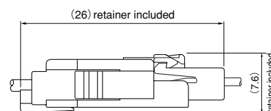
PAF Receptacle + PAL Receptacle
