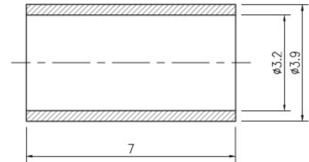
5.FERRULE
